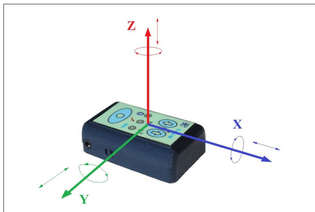
Рис. 2. Регистрирующее устройство инерционной безплатформенной системы. Показаны оси системы координат, по которым производится регистрация, как колебаний, так и вращений.
